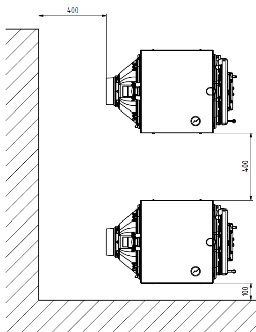
Rys. nr 5 Umiejscowienie kotła w kotłowni.
