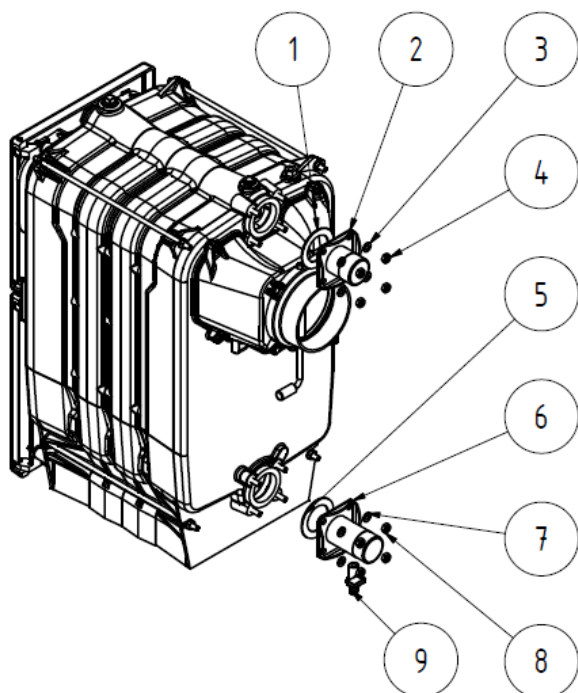
Rys. nr 6 Instalacja wymiennika kotłowego VIADRUS U 22 BASIC
