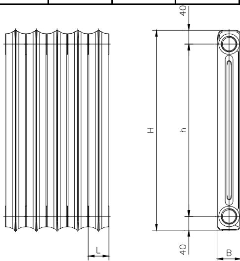
Rys. nr 2 Główne wymiary elementów Kalor 3
