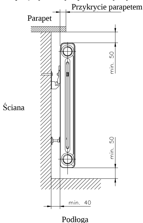
Rys. nr 3 Osadzanie grzejników Kalor 3
