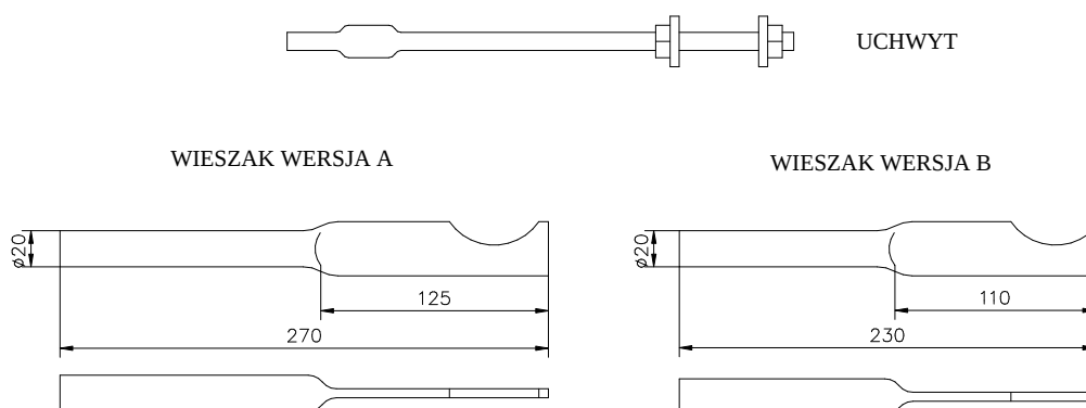
Rys. nr 3 Grzejnikowe wieszaki rurowe i uchwyt.
