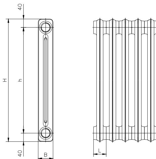
Rys. nr 2 Główne wymiary elementu Kalor
