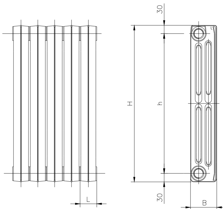
Rys. nr 2 Główne wymiary elementów Termo
