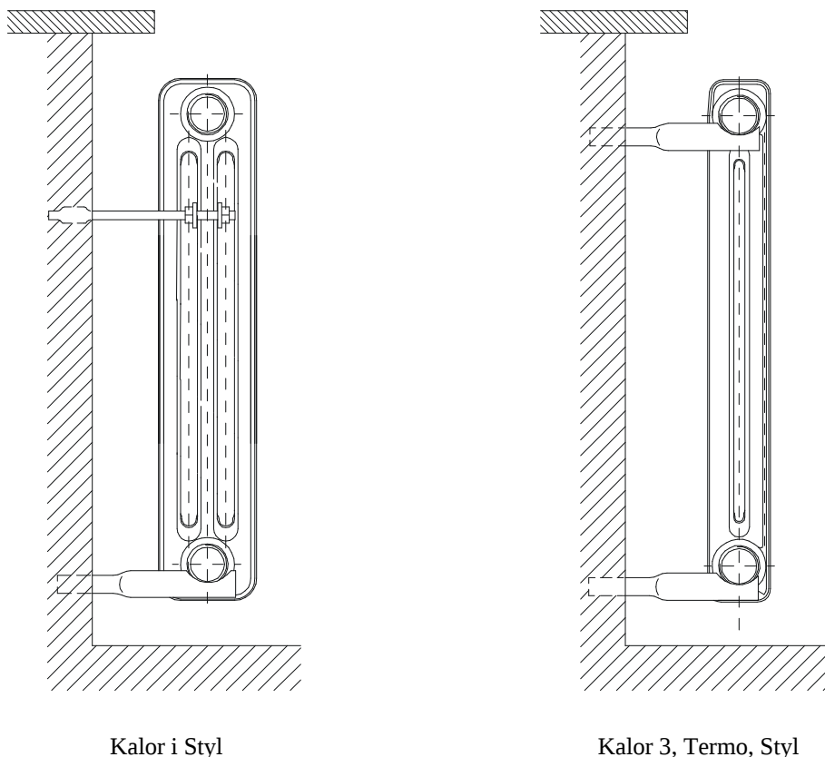
Rys. nr 2. Umocowanie grzejników za pomocą wieszaków rurowych i uchwytów.
