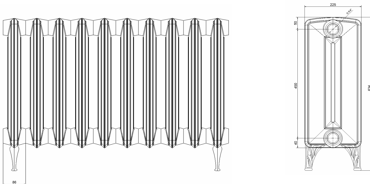
Rys. nr 2 Główne wymiary elementu BOHEMIA
