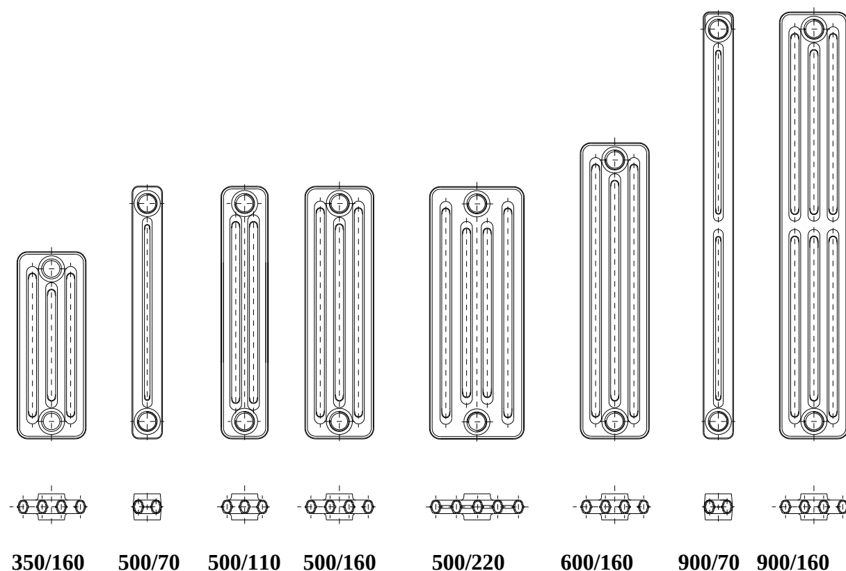
Rys. nr 1 Ogniwa grzewcze rodzaju Kalor
