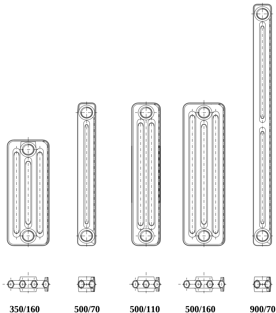
Rys. nr 1 Otopné články typu Kalor 3
