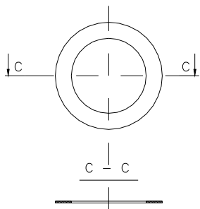
Uszczelka klimgeritowa pod korek 5/4"
