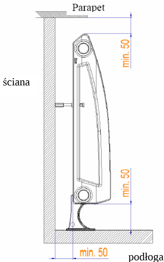
Rys. nr 3 Osadzanie grzejników STYL
