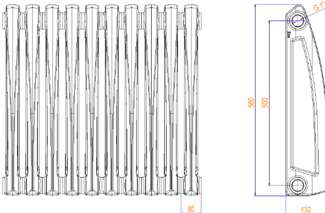
Rys. nr 2 Główne wymiary elementu STYL
