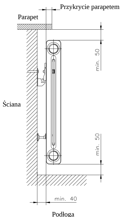
Rys. nr 3 Osadzanie grzejników Kolor
