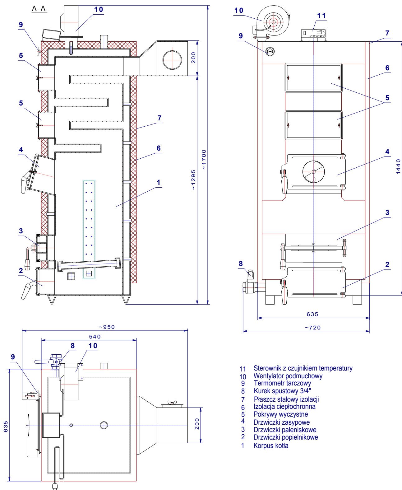
Rys.1 Schemat konstrukcyjny kotłów EN-ka Plus.
