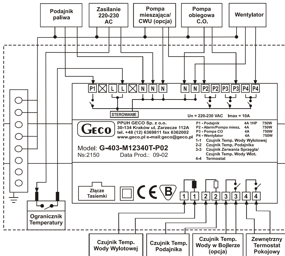
Rys. 2 Schemat podłączenia urządzeń i czujników do regulatora G-403-P02.
