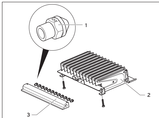
Rys. 6.8 Oznaczenie dysz
