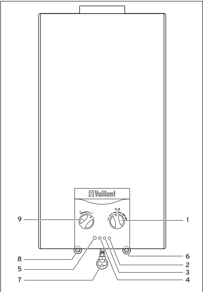
Rys. 4.1 Elementy obsługi
