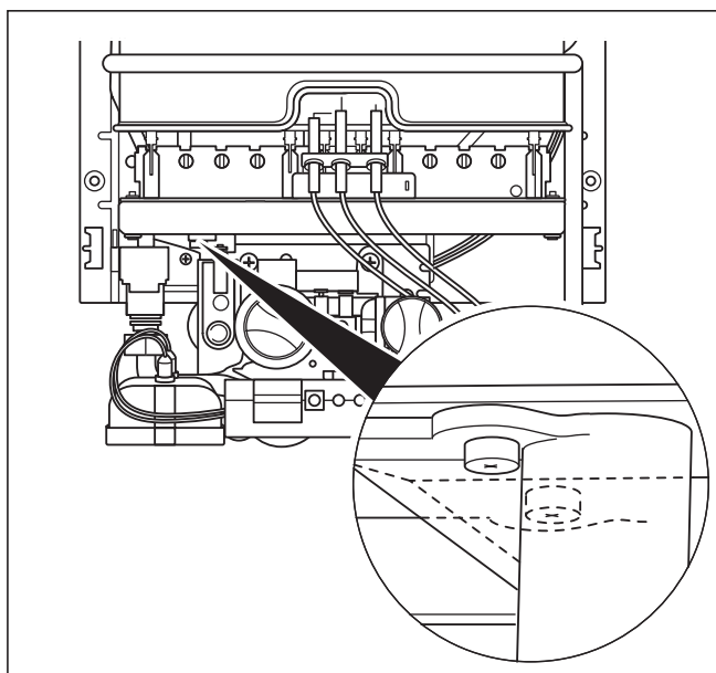
Rys. 7.3 Przymocowanie palnika do armatury gazowej - typ XI
