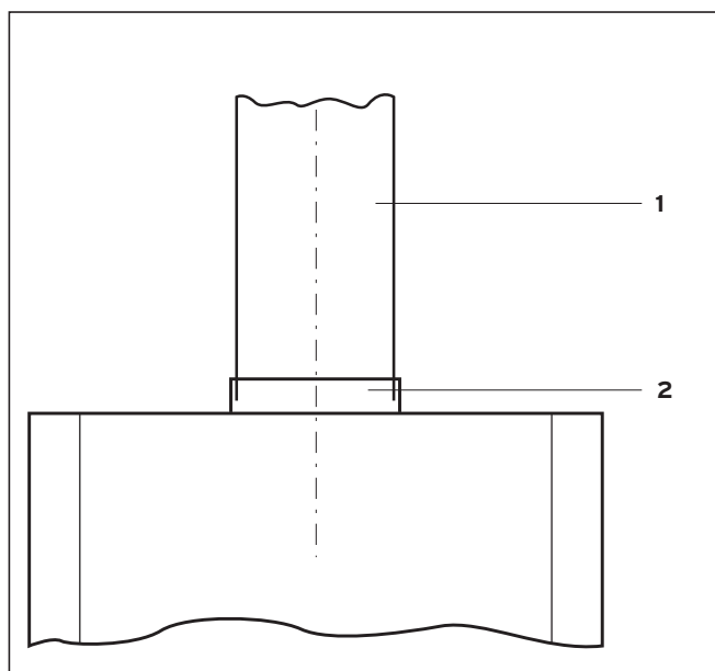
Rys. 5.1 Podłączanie do układu odprowadzania spalin
