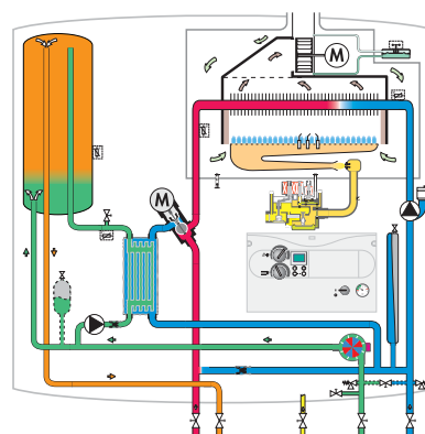
Pobór ciepłej wody (<8 l/min.) przy nagrzanim zasobnika.
