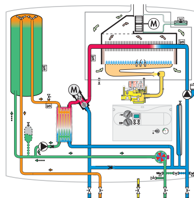
Ładowanie zasobnika bez poboru ciepłej wody.
